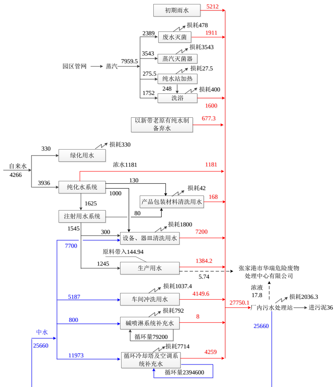
图 3.4-1 本项目水汽平衡图 (m³/a)
