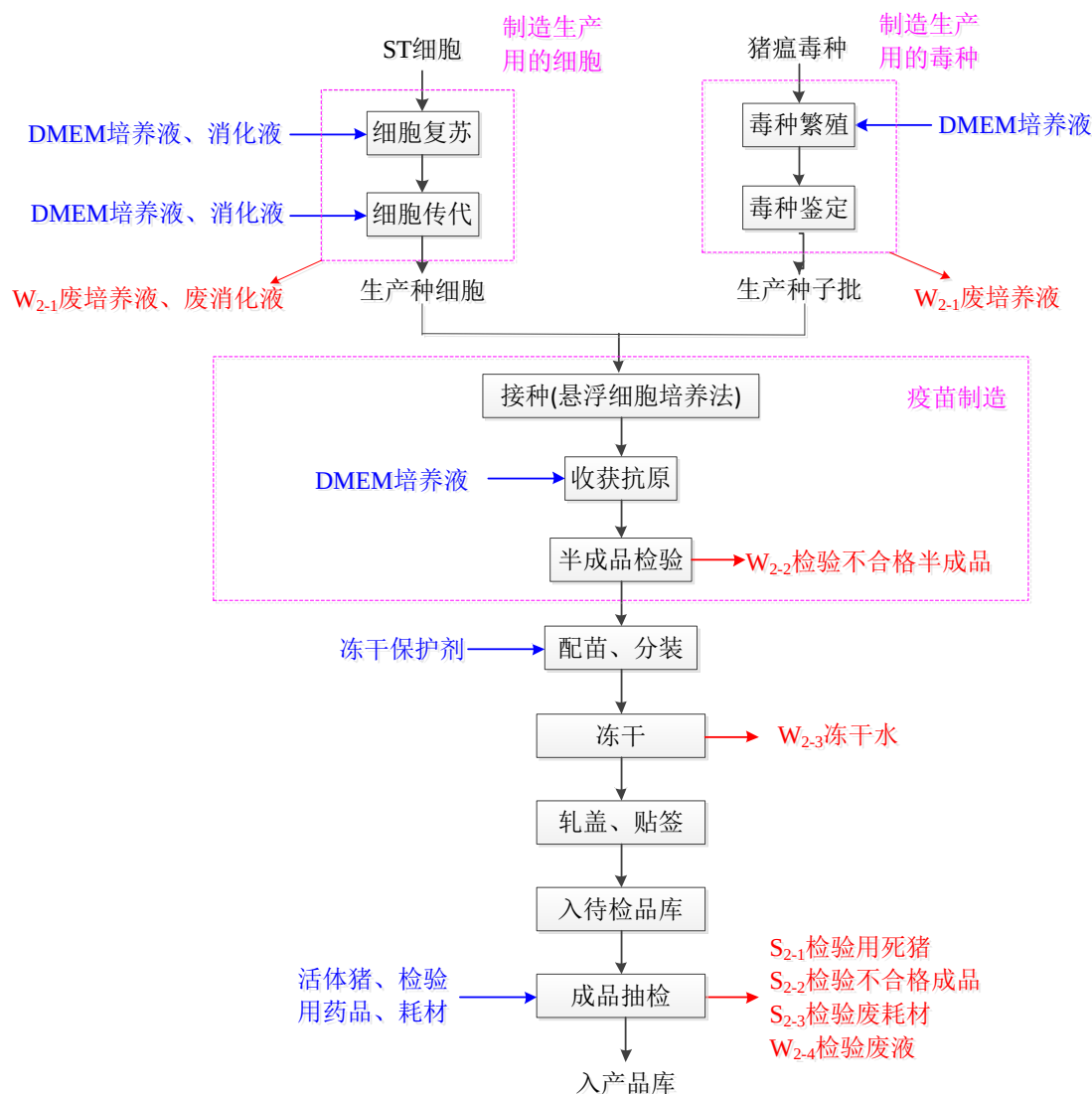
图 3.5-2 猪瘟活疫苗（传代细胞源）生产工艺流程图
