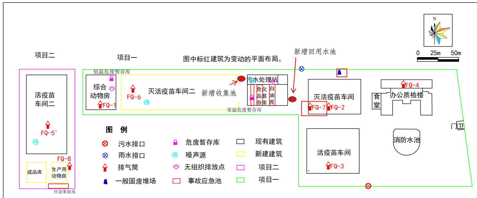
图 3.1-2 平面布置图
